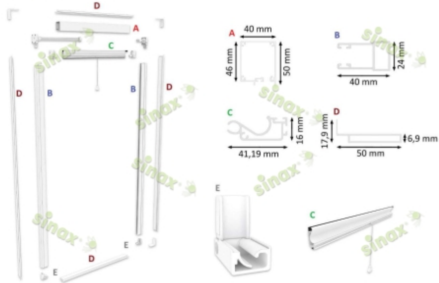
İÇTEN TAKMALI İDA STOR
