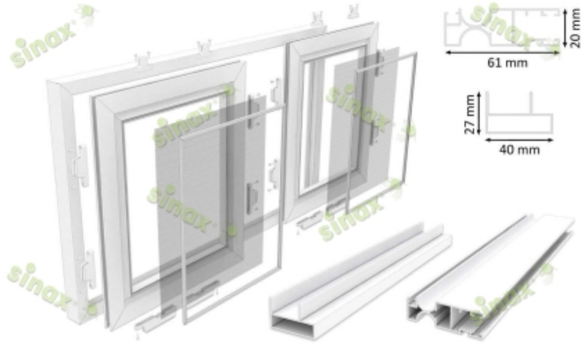
TUBA DELUXE SÜRME ÇİFT KANAT ÇİFTLİ RAY
