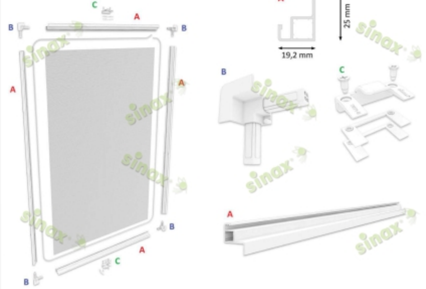
İÇTEN TAKMALI SABİT DELUXE
