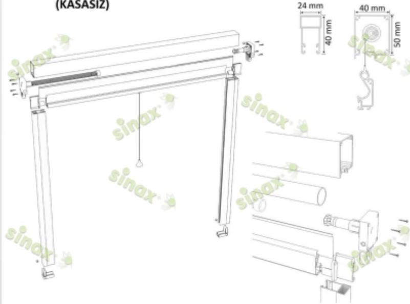
İDA 40 DİKEY STOR (KASASIZ)
