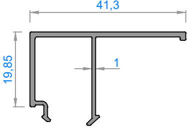
Sistem Kodu : 6155 Ağırlık (kg/mt): 0,310
