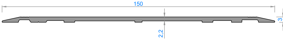
5306 - 0,905 kg/m
