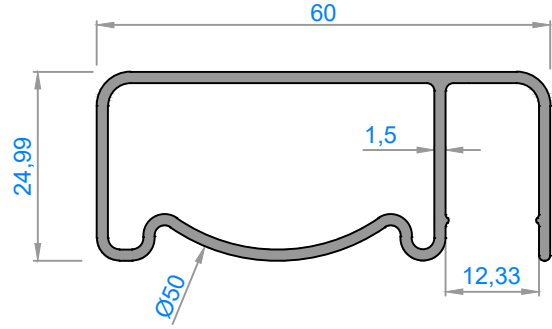
4003 - 0,720 kg/m
