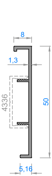
5434 - 0,245 kg/m
