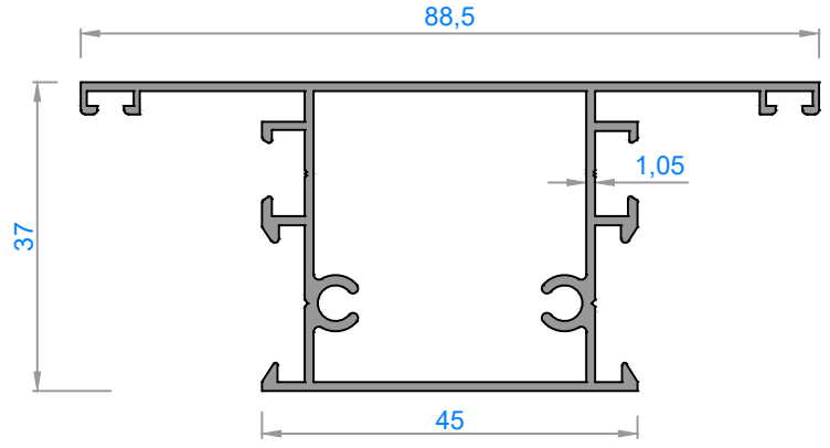
1306 - 0,810 kg/m
