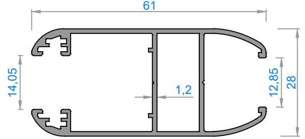
1312 - 0,670 kg/m
