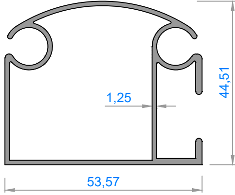
1190 - 0,824 kg/m
