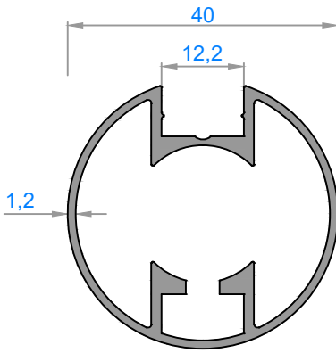
2384 - 0,640 kg/m
