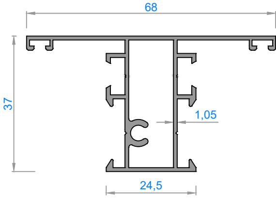
1307 - 0,665 kg/m
