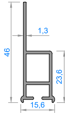
4402 - 0,347 kg/m
