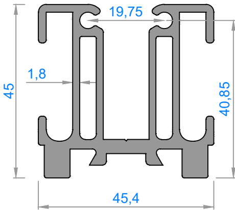
Sistem Kodu : FC50-6032 Ağırlık (kg/mt): 1,670
