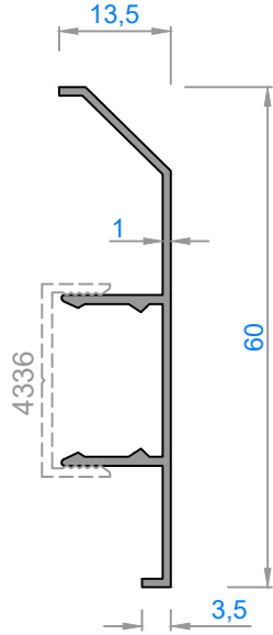
3918 - 0,272 kg/m
