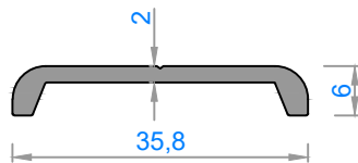
4536- 0,245 kg/m
