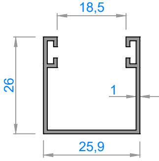
1099 - 0,259 kg/m
