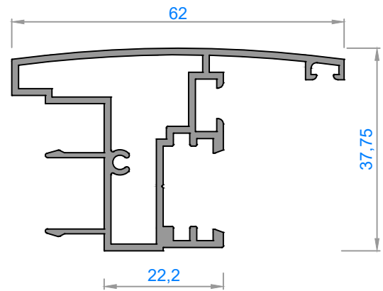
3008 - 0,805 kg/m
