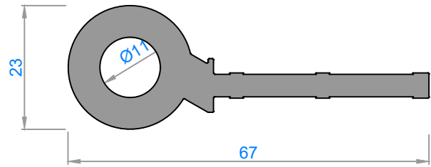
4530 - 1,435 kg/m
