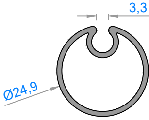
1734 - 0,323 kg/m
