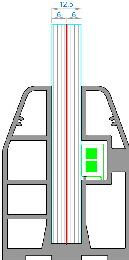
3929 - 2,971 kg/m
