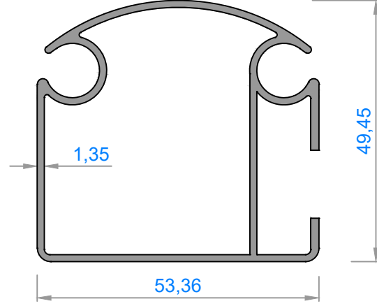
1230 - 0,810 kg/m
