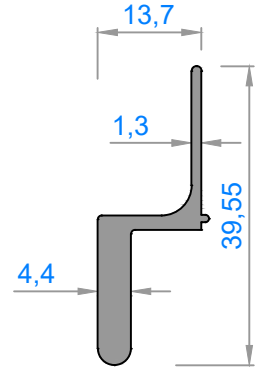
2099 - 0,407 kg/m
