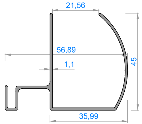
3587 - 0,493 kg/m
