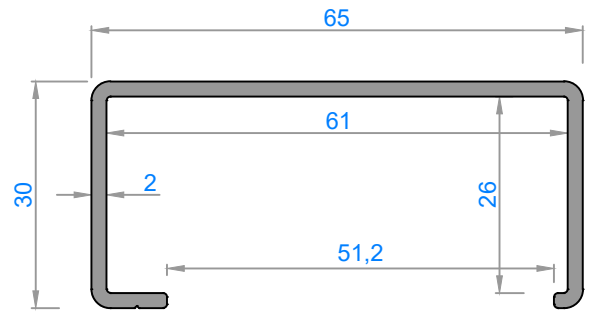
4340 - 0,694 kg/m
