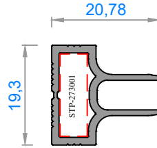
Sistem Kodu : FC50-6027 Ağırlık (kg/mt): 0,265 ( siyah eloksalı )
