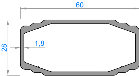
1360 - 0,910 kg/m
