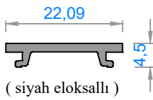
Sistem Kodu : FC50-6018
