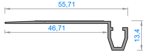
3921 - 0,240 kg/m
