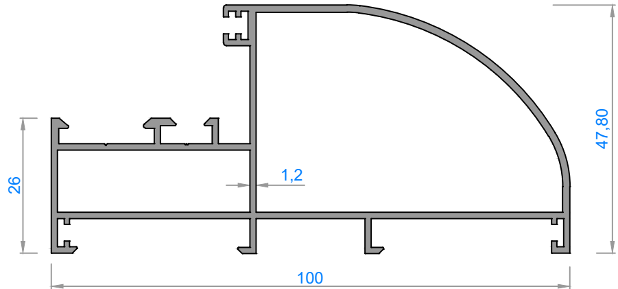
1325 - 1,190 kg/m
