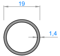
2140 - 0,211kg/m
