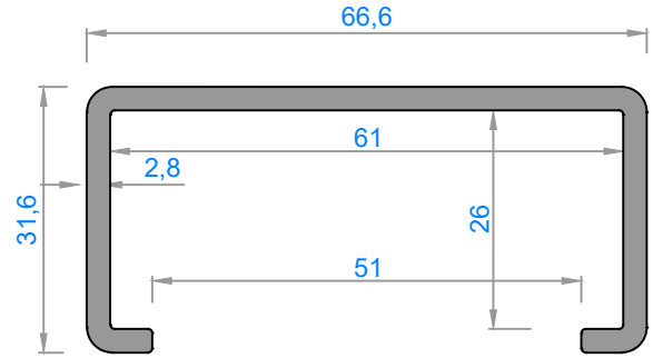
4293 - 0,997 kg/m
