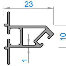
1242 - 0,250 kg/m
