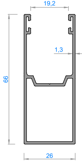
4729 - 0,700 kg/m
