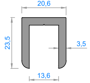
4321 - 0,560 kg/m
