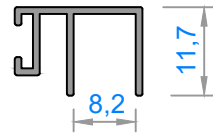
4231 - 0,126 kg/m
