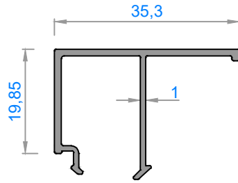
Sistem Kodu : 6158 Ağırlık (kg/mt): 0,289
