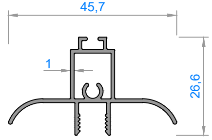
4398 - 0,334 kg/m
