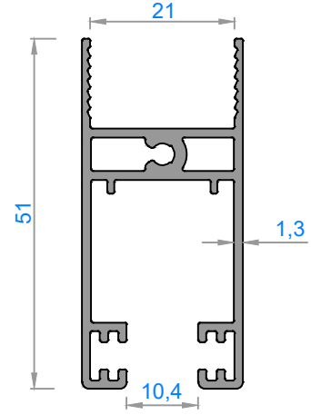
6205 - 0,650 kg/m
