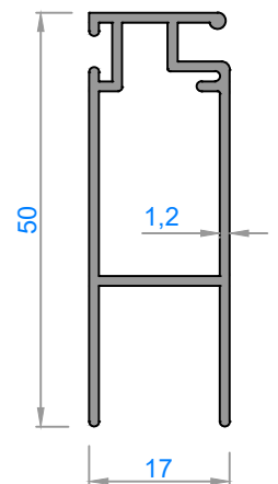
4867 - 0,470 kg/m
