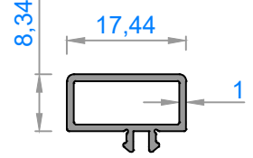
Sistem Kodu : FC50-6028 Ağırlık (kg/mt): 0,145
