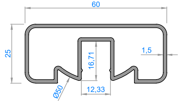
3955 - 0,827 kg/m
