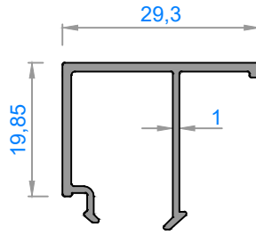
Sistem Kodu : 6161 Ağırlık (kg/mt): 0,268
