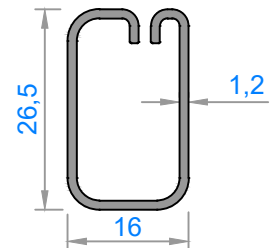
4400 - 0,255 kg/m
