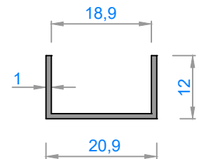
4407 - 0,116 kg/m
