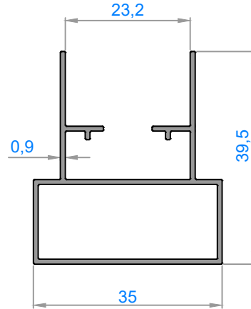
4473 - 0,397 kg/m
