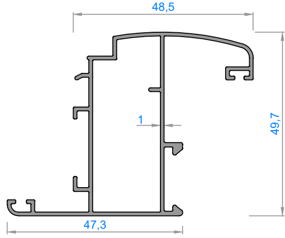
3462 - 0,672 kg/m
