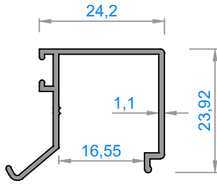
4094 - 0,244 kg/m
