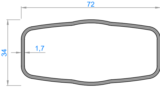
2101 - 0,845 kg/m
