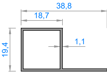
2076 - 0,260 kg/m
