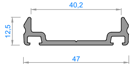
Sistem Kodu : FC50-6022
