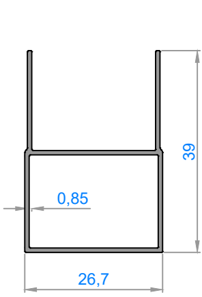
4464 - 0,295 kg/m
