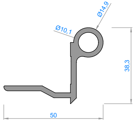
4535- 0,718 kg/m
