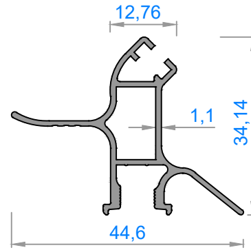
1732 - 0,383 kg/m
