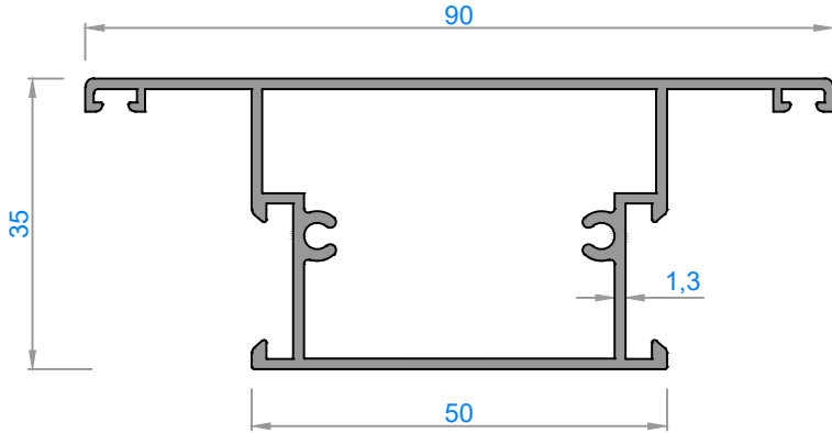
3007 - 0,895 kg/m
