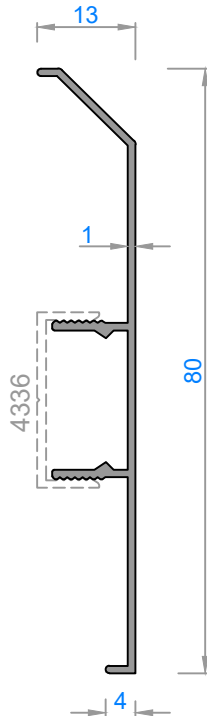
4346 - 0,313 kg/m
