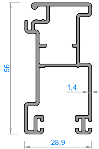
4731 - 0,800 kg/m
