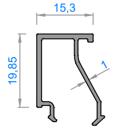
Sistem Kodu : 6168 Ağırlık (kg/mt): 0,222
