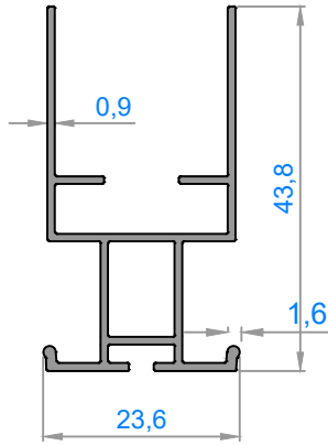
4465 - 0,375 kg/m
