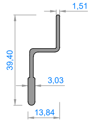
1142 - 0,407 kg/m
