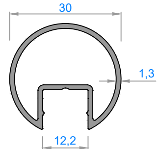
3580 - 0,400 kg/m
