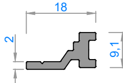
Sistem Kodu : FC50-6019
