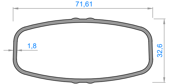
1511 - 0,865 kg/m
