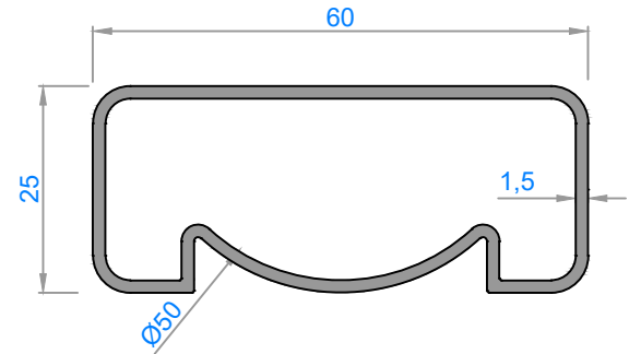
3561 - 0,718 kg/m
