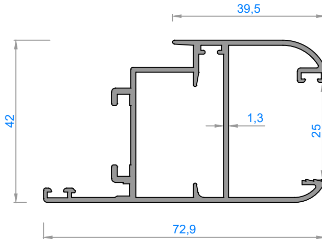
3057 - 0,935 kg/m
