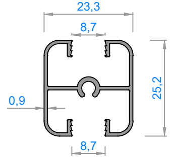
4050 - 0,285 kg/m
