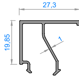
Sistem Kodu : 6162 Ağırlık (kg/mt): 0,264
