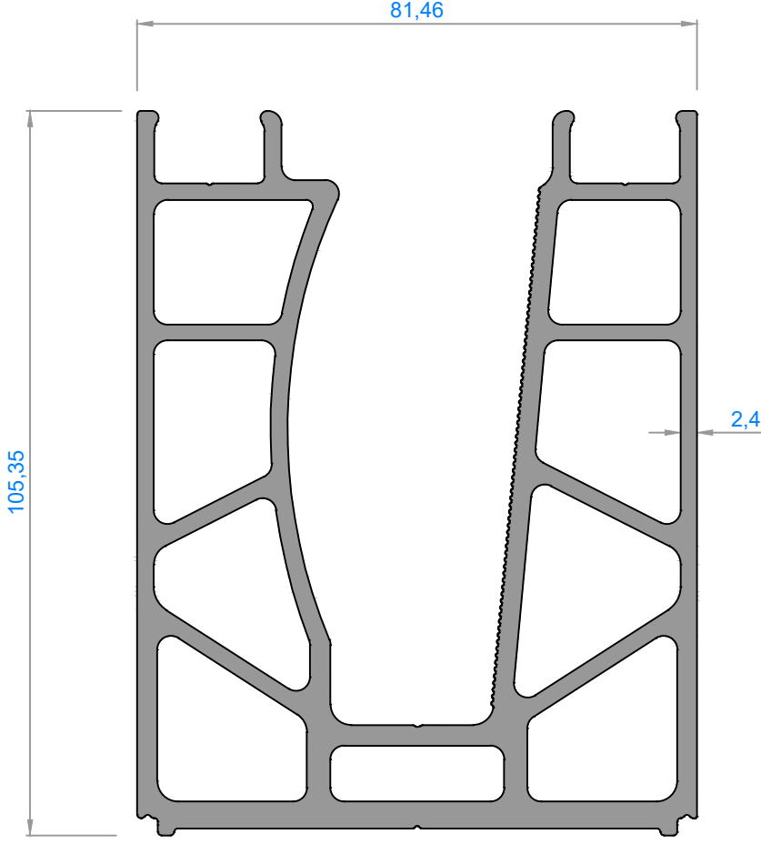
4800 - 5,322 kg/m
