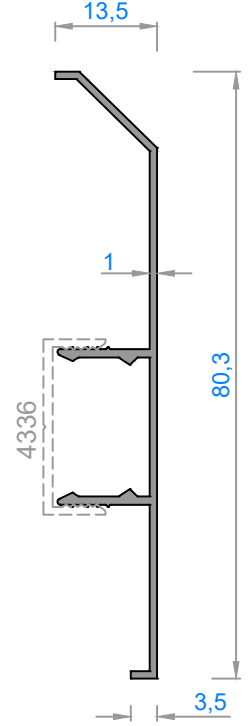
3919 - 0,330 kg/m
