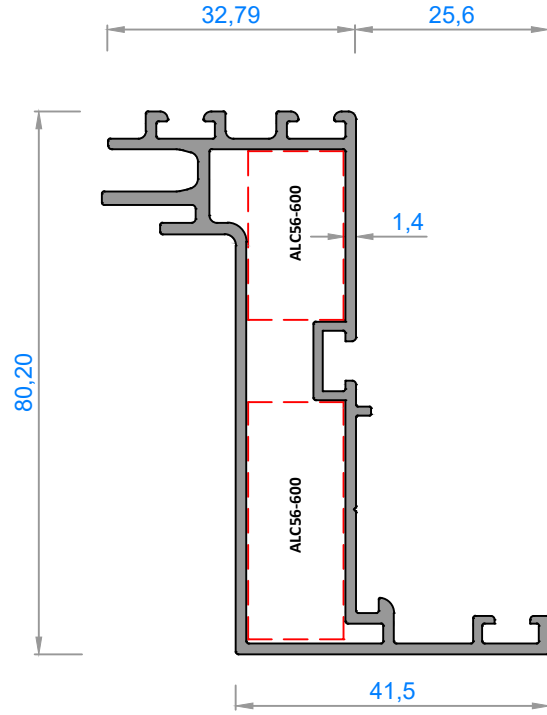
Sistem Kodu : FC50-6013
