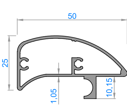
1879 - 0,569 kg/m
