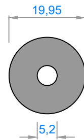
4364 - 0,789 kg/m
