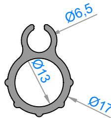
5126 - 0,343 kg/m
