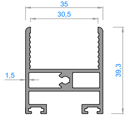
4379 - 0,794 kg/m 4379 - 4378 ile beraber çalışmaktadır.
