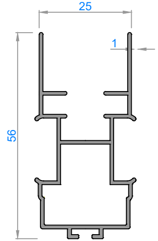
4474 - 0,395 kg/m
