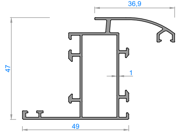
5386 - 0,735 kg/m
