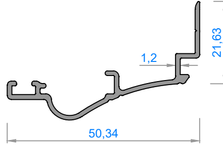
Sistem Kodu : ALC56-500 Ağırlık (kg/mt): 0,325
