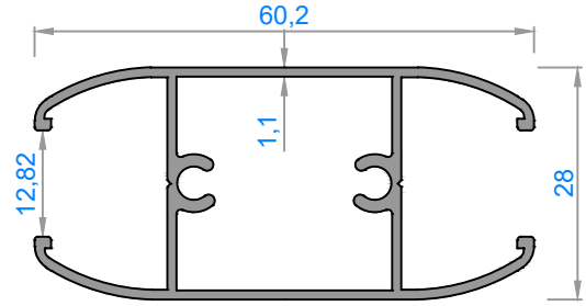
1314 - 0,658 kg/m
