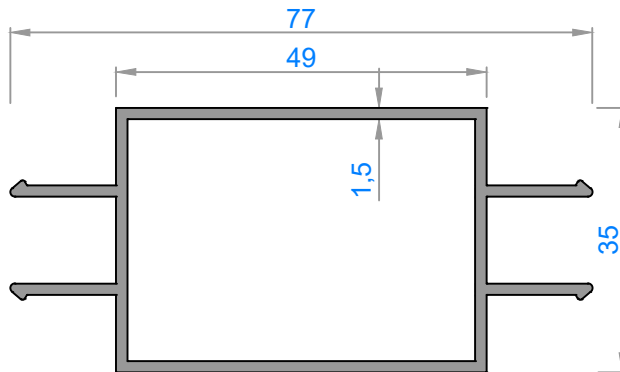
1381 - 0,890 kg/m
