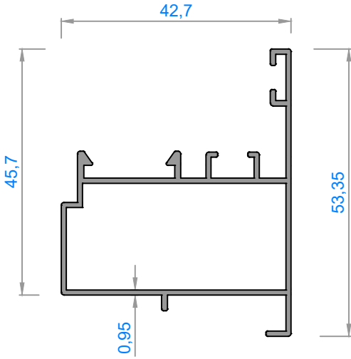
2600 - 0,520 kg/m
