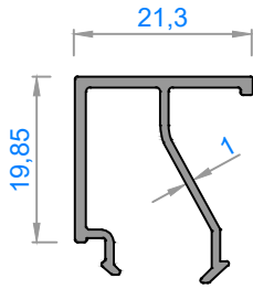
Sistem Kodu : 6165 Ağırlık (kg/mt): 0,243
