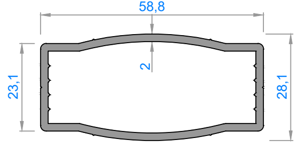
1195 - 0,855 kg/m
