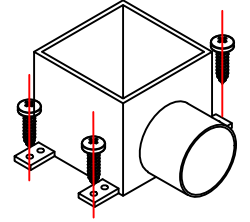
FC50-160 ALÜMİNYUM DİREK PAPUCU ALUMINUM POLE LUGS
