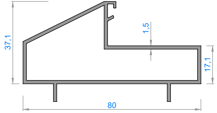
2640 - 0,965 kg/m
