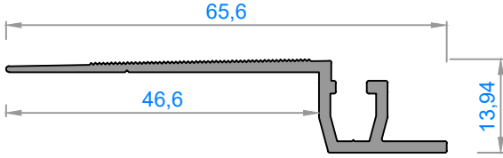
3914 - 0,370 kg/m
