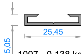
1097 - 0,138 kg/m
