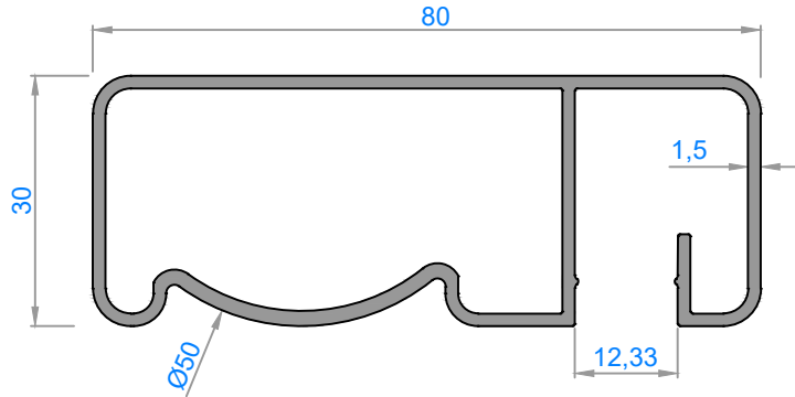
3816 - 1,012 kg/m
