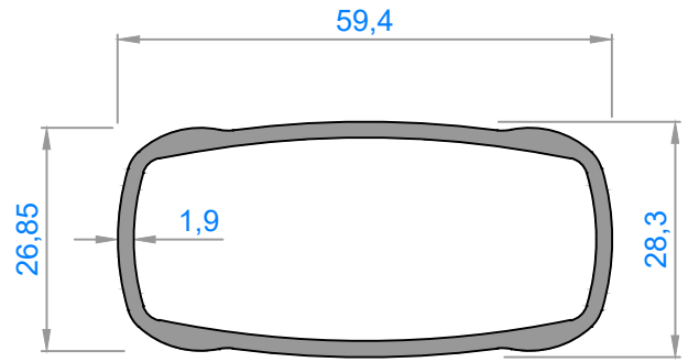
1885 - 0,840 kg/m
