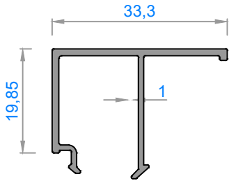
Sistem Kodu : 6159 Ağırlık (kg/mt): 0,282
