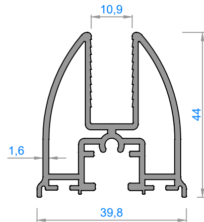
* 4122 - 1,005 kg/m
