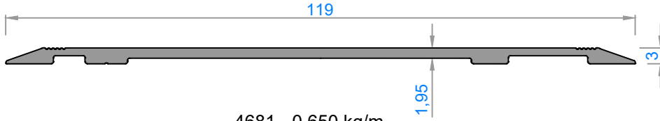
4681 - 0,650 kg/m
