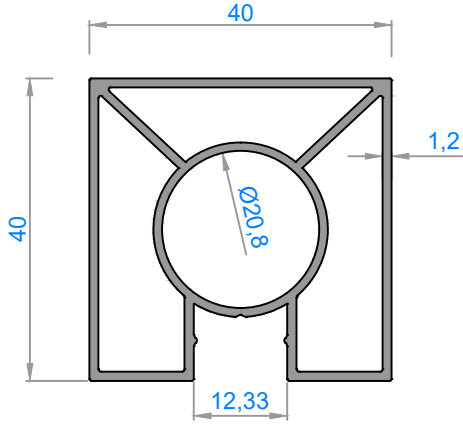
3818 - 0,874 kg/m
