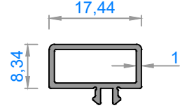
Sistem Kodu : FC50-6028 Ağırlık (kg/mt): 0,145
