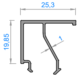
Sistem Kodu : 6163 Ağırlık (kg/mt): 0,257
