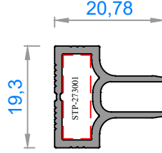
Sistem Kodu : FC50-6027 Ağırlık (kg/mt): 0,265 ( siyah e oksallı )
