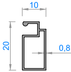
1727 - 0,143 kg/m
