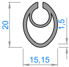
1192 - 0,263 kg/m
