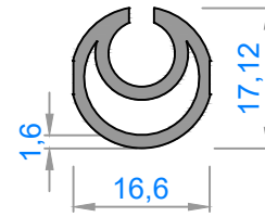
1191 - 0,293 kg/m
