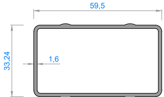
1189 - 0,795 kg/m
