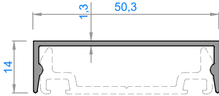
Sistem Kodu : FC50-6024 Ağırlık (kg/mt): 0,290
