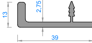
4613 - 0,455 kg/m
