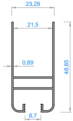
4048 - 0,384 kg/m
