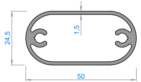
3849 - 0,699 kg/m
