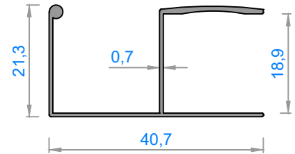
4427 - 0,219 kg/m
