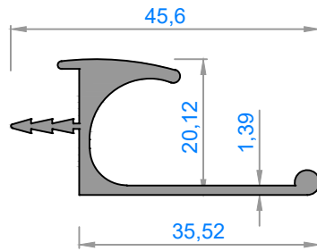
2508 - 0,428 kg/m
