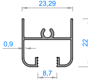
4049 - 0,231 kg/m
