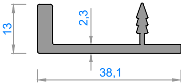
3326 - 0,409 kg/m
