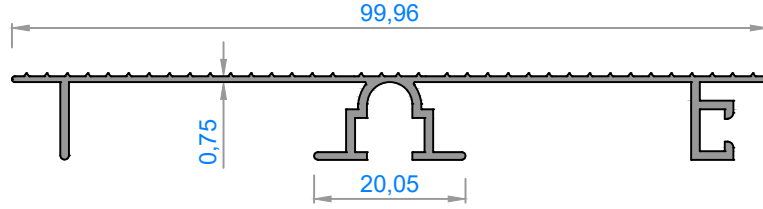
2534 - 0,429 kg/m
