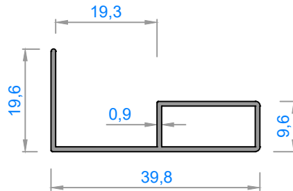
4450 - 0,228 kg/m
