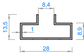
4551 - 0,190 kg/m
