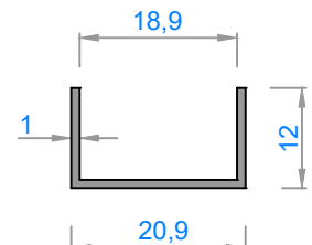
4407 - 0,116 kg/m
