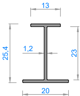
4745 - 0,182 kg/m
