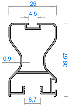
4053 - 0,395 kg/m
