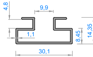
1947 - 0,257 kg/m
