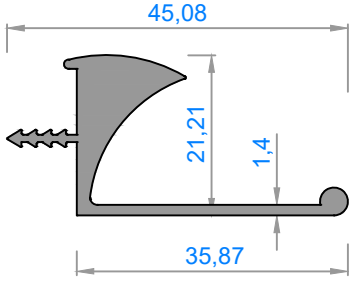
2207 - 0,526 kg/m
