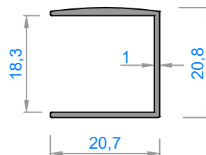
4429 - 0,167 kg/m
