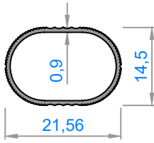
4411 - 0,126 kg/m
