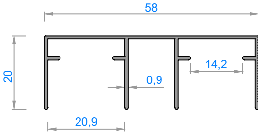
4444 - 0,357 kg/m
