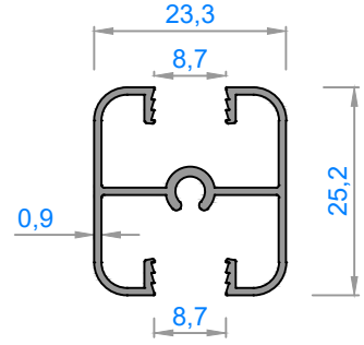
4050 - 0,285 kg/m
