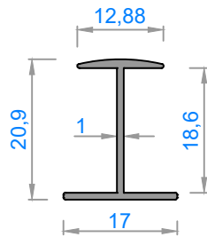
4428 - 0,133 kg/m
