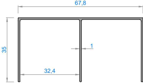
4051 - 0,460 kg/m
