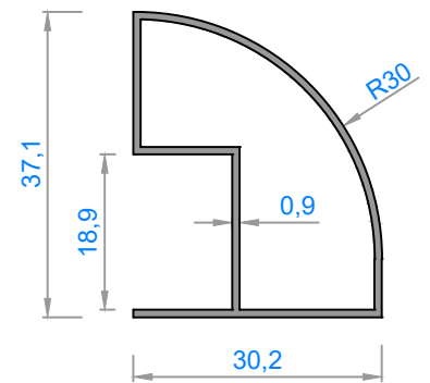
4435 - 0,318 kg/m
