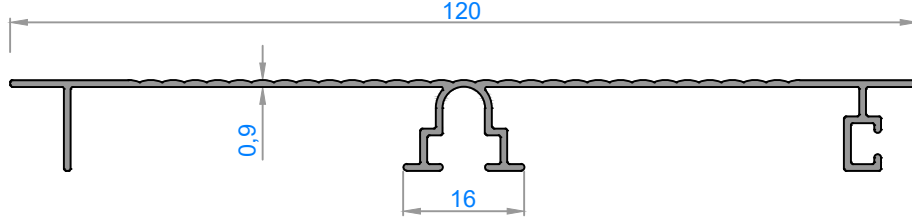
3070 - 0,436 kg/m
