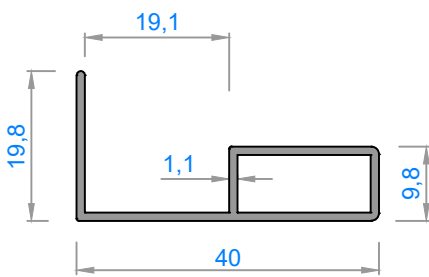
4406 - 0,278 kg/m
