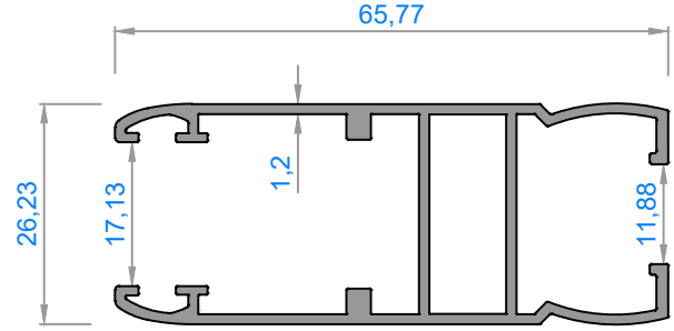
4084 - 0,747 kg/m
