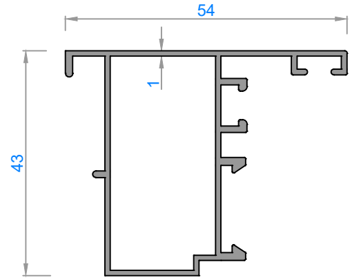
4089 - 0,575 kg/m
