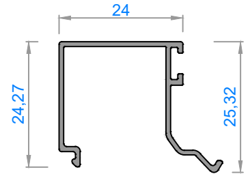
5385 - 0,220 kg/m
