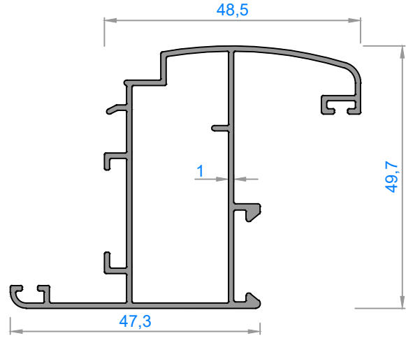
3462 - 0,672 kg/m
