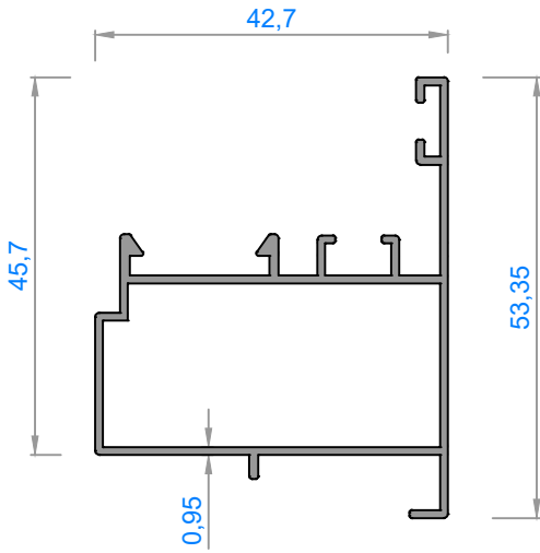
2600 - 0,520 kg/m
