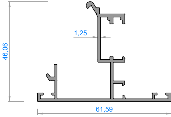
4083 - 0,640 kg/m
