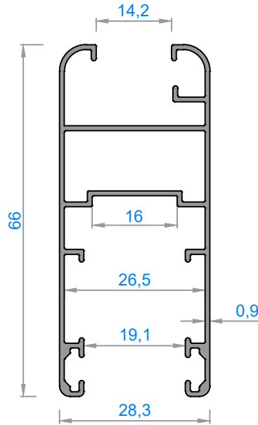
3564 - 0,610 kg/m
