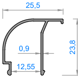
3463 - 0,173 kg/m
