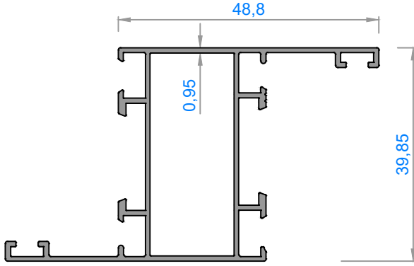
4092 - 0,564 kg/m
