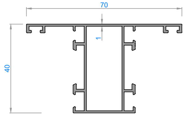
4091 - 0,634 kg/m
