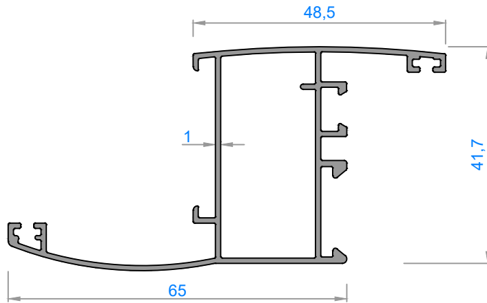
3465 - 0,691 kg/m
