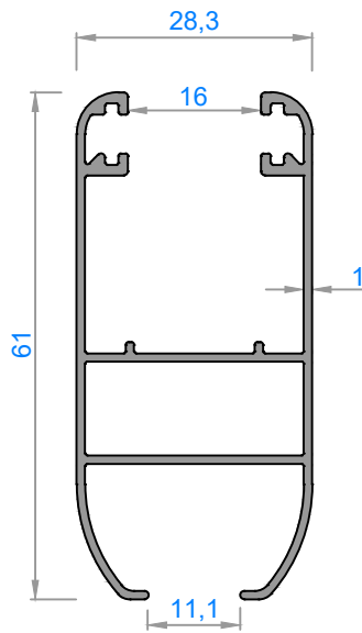
3459 - 0,590 kg/m
