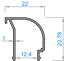
2602 - 0,190 kg/m
