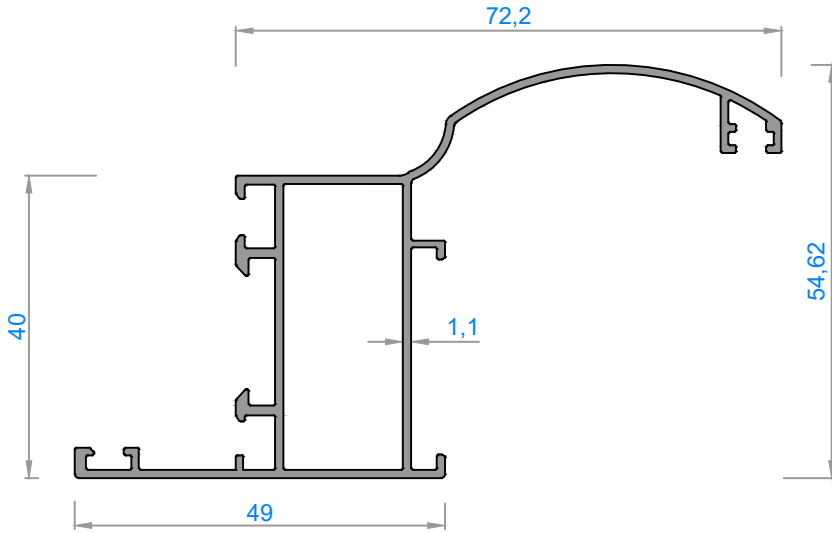
5387 - 0,770 kg/m
