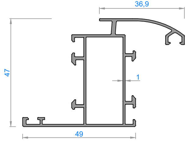
5386 - 0,735 kg/m
