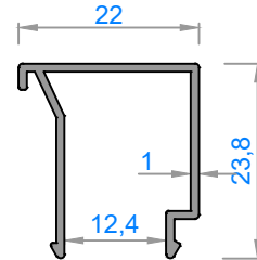
2603 - 0,200 kg/m
