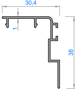
3461 - 0,235 kg/m
