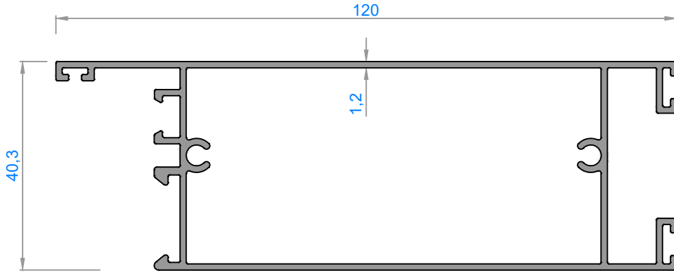
3458 - 1,238 kg/m
