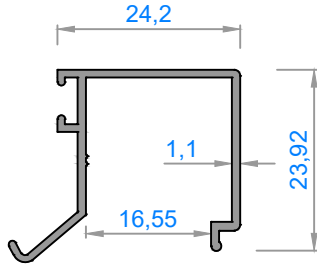
4094 - 0,244 kg/m
