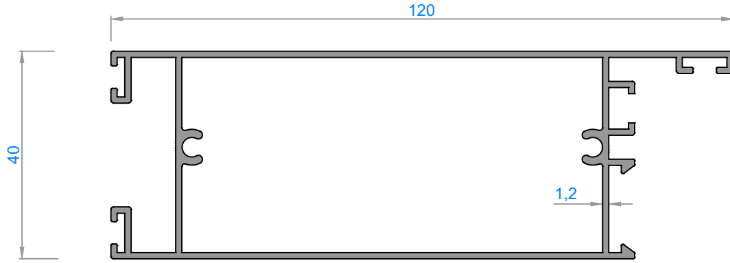
2599 - 1,230 kg/m
