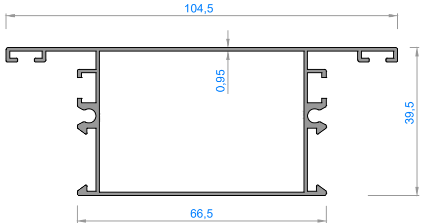
2598 - 0,848 kg/m
