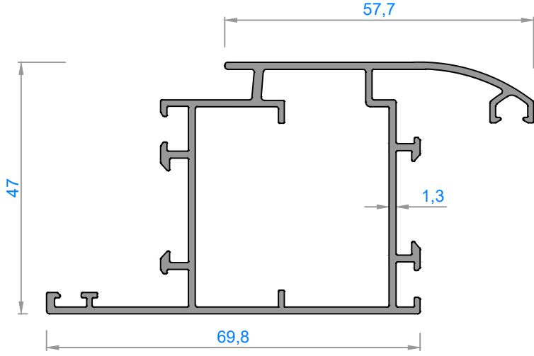
5388 - 1,070 kg/m
