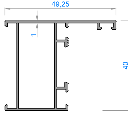
4093 - 0,504 kg/m
