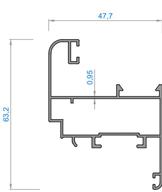
2595 - 0,643 kg/m
