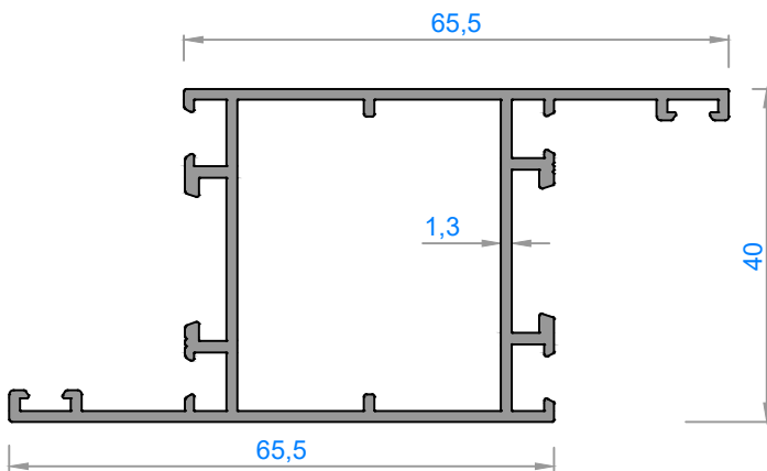
4090 - 0,931 kg/m
