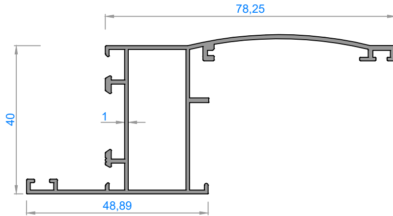
4096 - 0,742 kg/m
