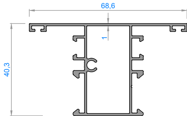
3460 - 0,696 kg/m
