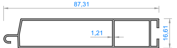
1503 - 0,642 kg/m
