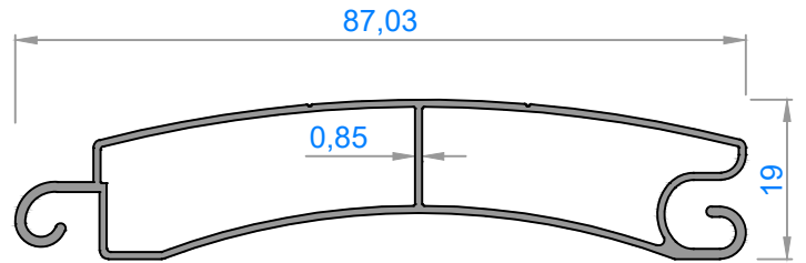
1507 - 0,555 kg/m
