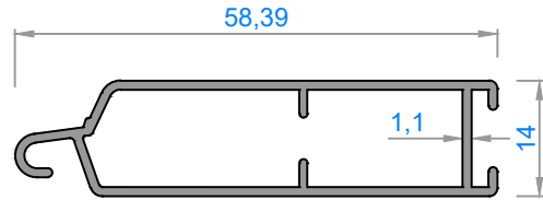
3050 - 0,435 kg/m
