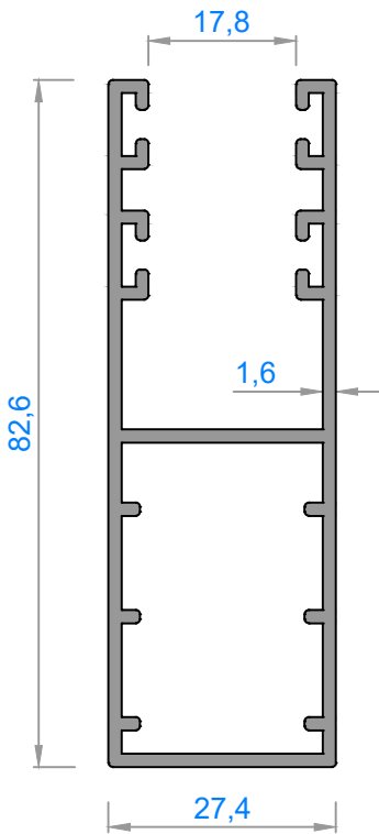
3396 - 1,155 kg/m
