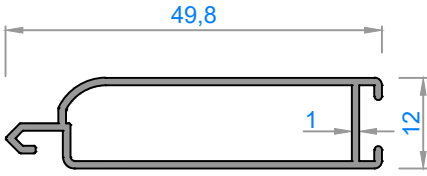
3137 - 0,320 kg/m
