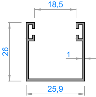
1099 - 0,259 kg/m
