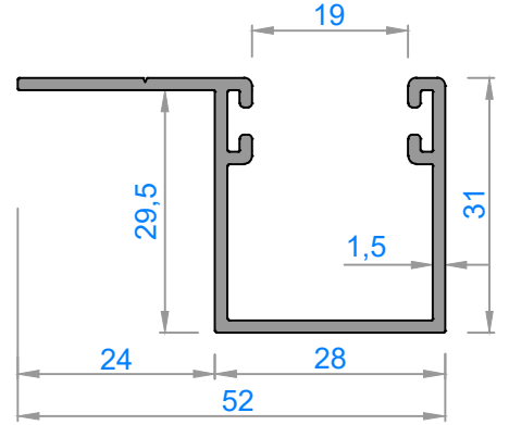
2317 - 0,531 kg/m
