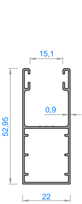
2255 - 0,430 kg/m
