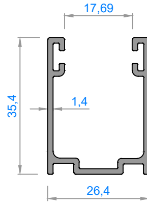
4727 - 0,455 kg/m
