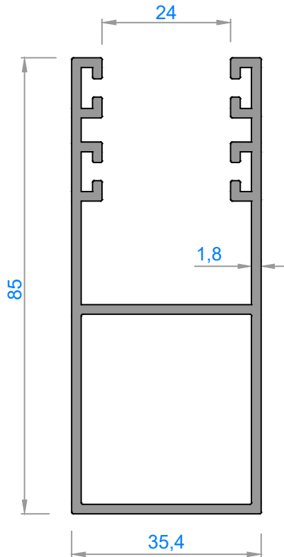
1501- 1,375 kg/m
