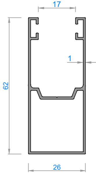
4730 - 0,555 kg/m
