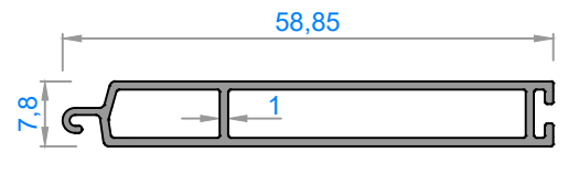
3376 - 0,366 kg/m
