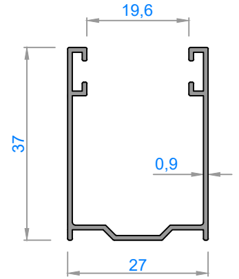
3888 - 0,292 kg/m
