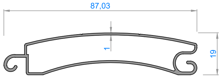
1505 - 0,607 kg/m
