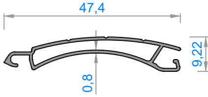
3097 - 0,232 kg/m
