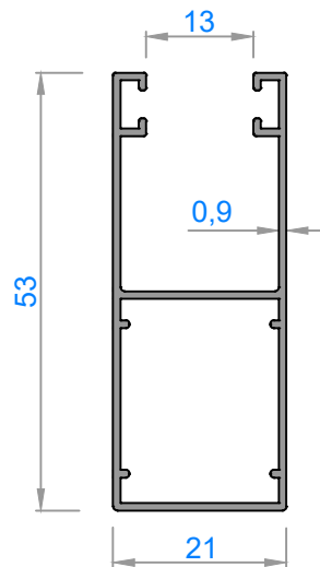
3885 - 0,405 kg/m
