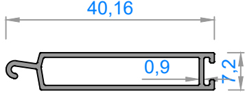
3626 - 0,222 kg/m
