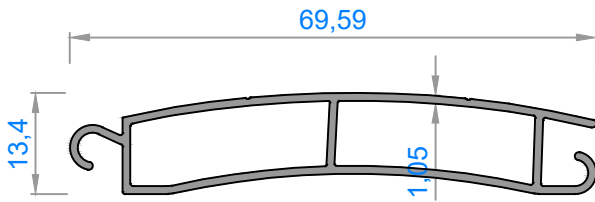
2455 - 0,480 kg/m
