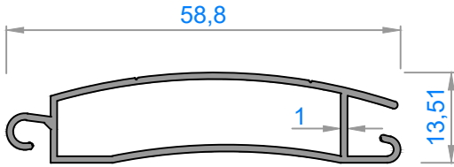
1504 - 0,378 kg/m
