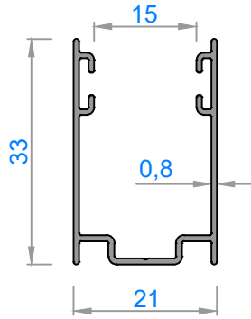
3334 - 0,240 kg/m
