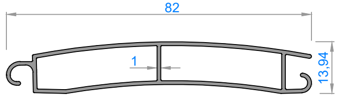
3254 - 0,532 kg/m
