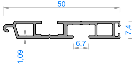
4728 - 0,350 kg/m
