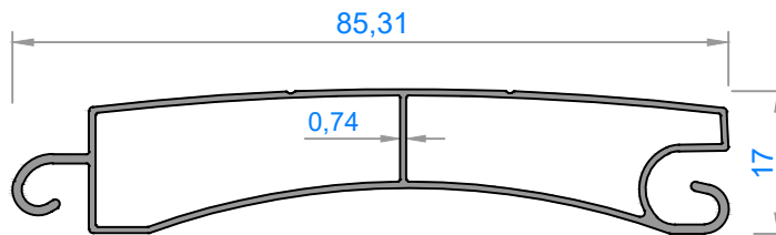
4227 - 0,490 kg/m
