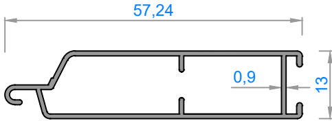
3891 - 0,347 kg/m
