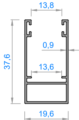
3624 - 0,315 kg/m
