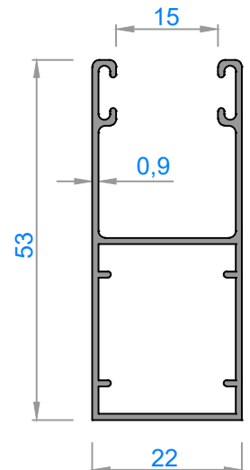
3059 - 0,420 kg/m
