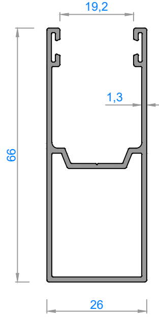
4729 - 0,700 kg/m
