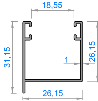
2161 - 0,263 kg/m
