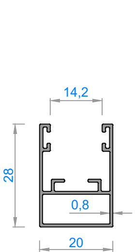
3625 - 0,265 kg/m
