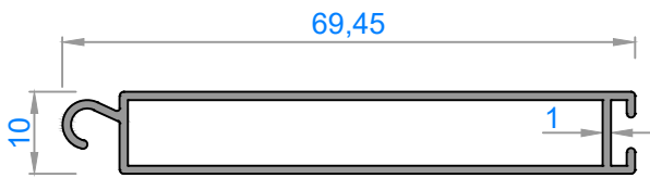
2588 - 0,428 kg/m
