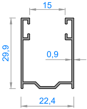
3884 - 0,245 kg/m
