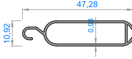
2162 - 0,280 kg/m
