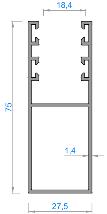
1500 - 0,910 kg/m
