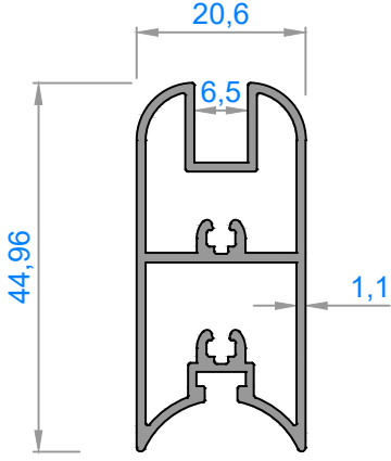
3390 - 0,579 kg/m
