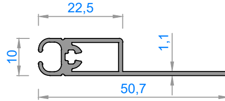
1246 - 0,318 kg/m
