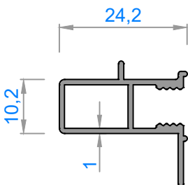
1473 - 0,236 kg/m
