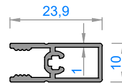
1729 - 0,220 kg/m
