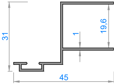
1492 - 0,285 kg/m
