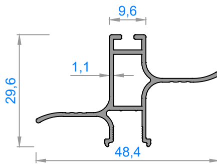
1731 - 0,347 kg/m
