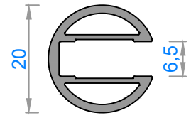
3392 - 0,295 kg/m
