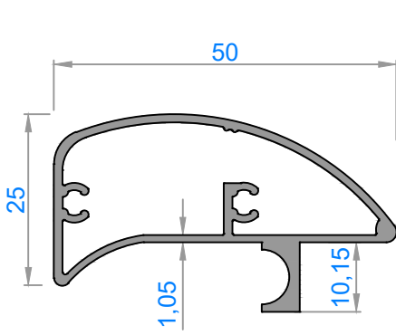
1879 - 0,569 kg/m
