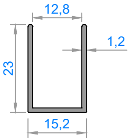
4399 - 0,190 kg/m
