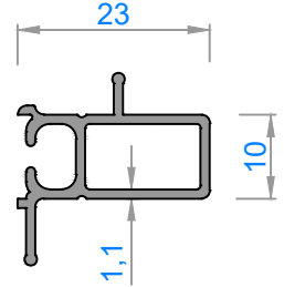
1176 - 0,247 kg/m
