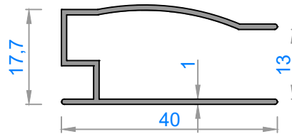
3126 - 0,276 kg/m
