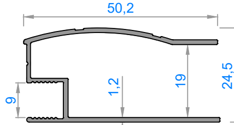
3450 - 0,403 kg/m
