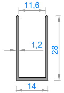
1234 - 0,220 kg/m
