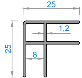
3637 - 0,307 kg/m
