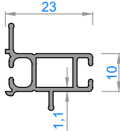
1244 - 0,258 kg/m
