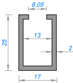
4169 - 0,368 kg/m
