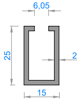
4125 - 0,357 kg/m
