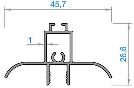
4398 - 0,334 kg/m
