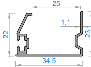
1237 - 0,298 kg/m
