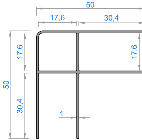
3636 - 0,528 kg/m
