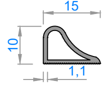
3586 - 0,113 kg/m
