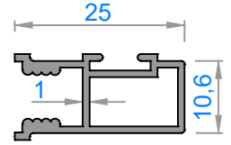
1494 - 0,300 kg/m
