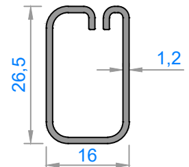
4400 - 0,255 kg/m
