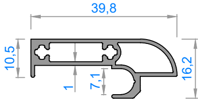
3123 - 0,368 kg/m
