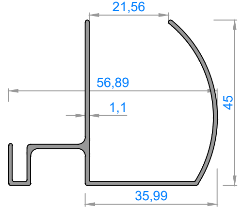
3587 - 0,493 kg/m
