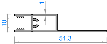
1472 - 0,273 kg/m
