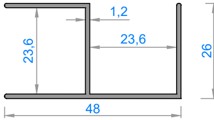
1236 - 0,391 kg/m
