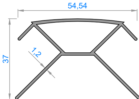
2531 - 0,570 kg/m
