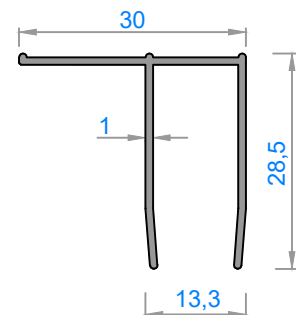
4818 - 0,230 kg/m
