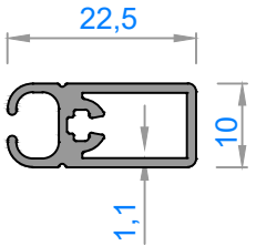
1730 - 0,231 kg/m
