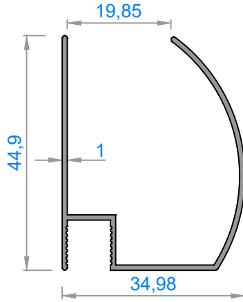
2904 - 0,352 kg/m
