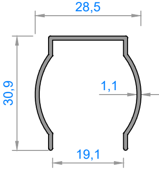
4394 - 0,250 kg/m
