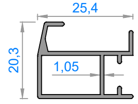
1238 - 0,274 kg/m
