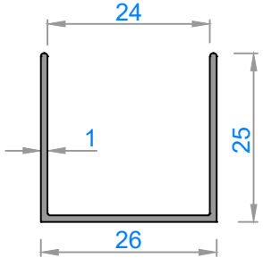
1695 - 0,201 kg/m
