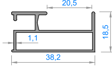
4396 - 0,381 kg/m
