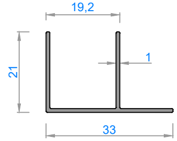
4795 - 0,197 kg/m
