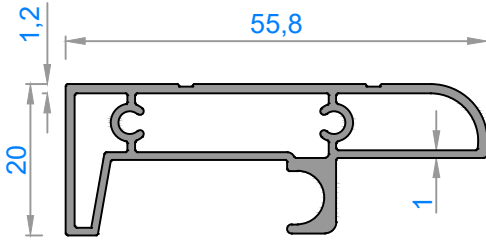
3451 - 0,577 kg/m
