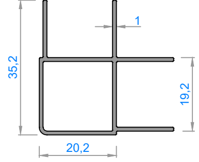
4798 - 0,369 kg/m
