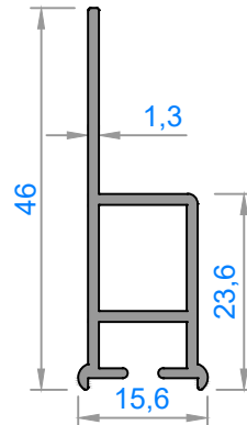
4402 - 0,347 kg/m
