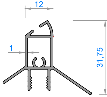
4397 - 0,338 kg/m
