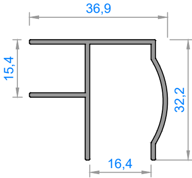
4401 - 0,363 kg/m
