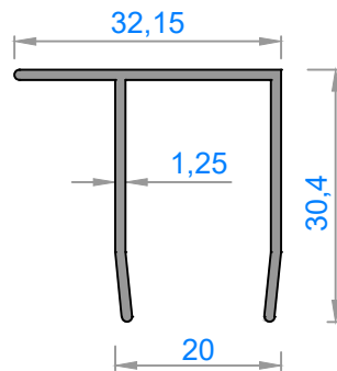
1958 - 0,248 kg/m
