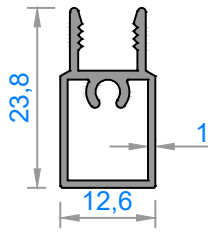
4395 - 0,228 kg/m
