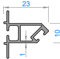
1732 - 0,383 kg/m
