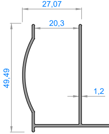
3391 - 0,423 kg/m
