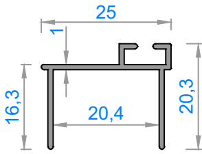
1206 - 0,187 kg/m
