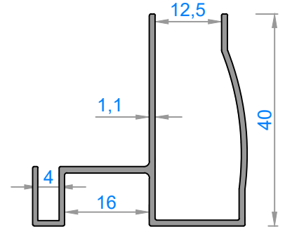
4267 - 0,411 kg/m
