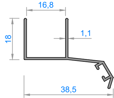
4403 - 0,250 kg/m
