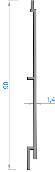
1084 - 0,400 kg/m
