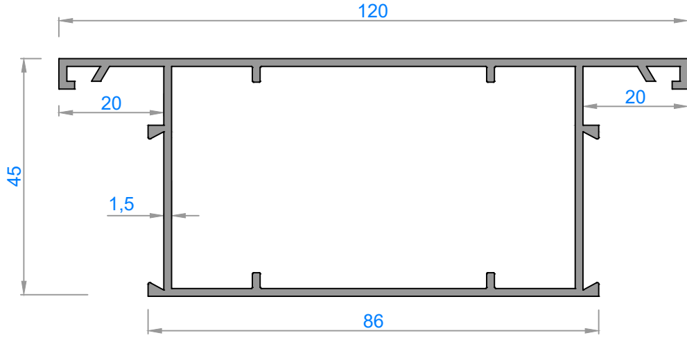
1103 - 1,343 kg/m
