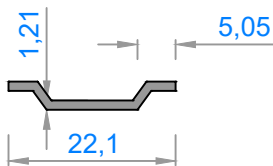
1098 - 0,081 kg/m
