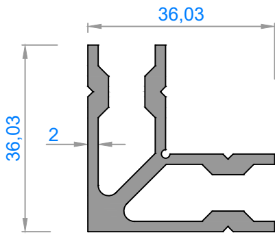
1088 - 0,948 kg/m
