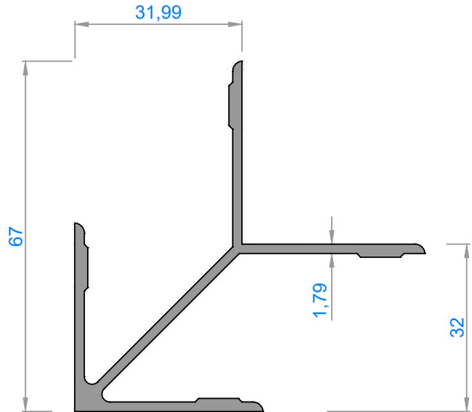
1089 - 0,953 kg/m
