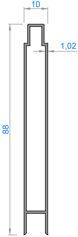
1083 - 0,540 kg/m
