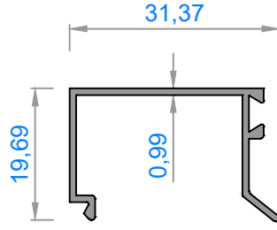
1081 - 0,209 kg/m
